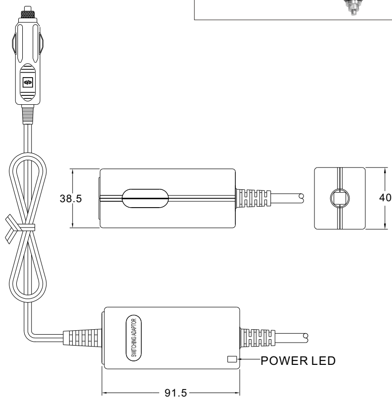
UNIT:mm
