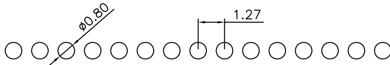
P.C.B LAYOUT
