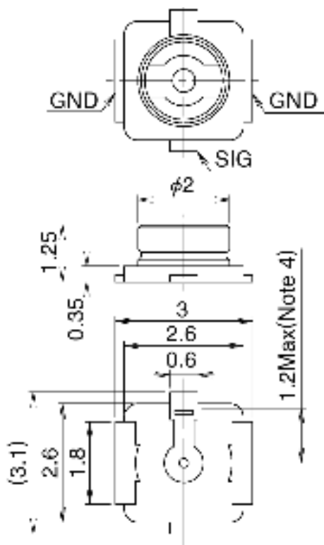
U.FL-R-SMT-1
