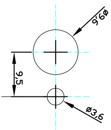
轴端安装尺寸
