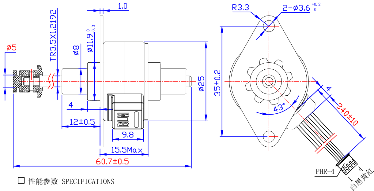
□ 外形图 DIMENSIONS (unit=mm)
