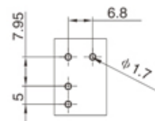
P.C.B. LAYOUT(1:1)
