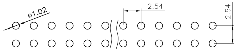
P.C.B LAYOUT
