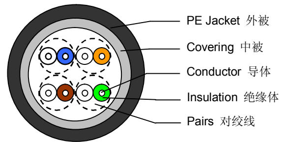
UTP 线材结构图
