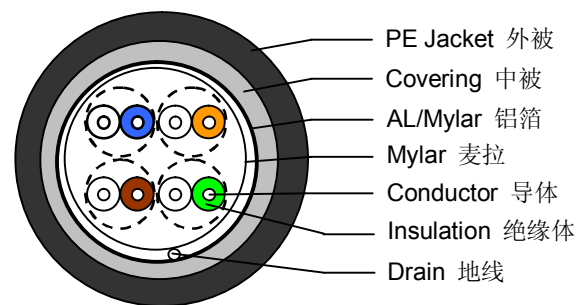
FTP 线材结构图
