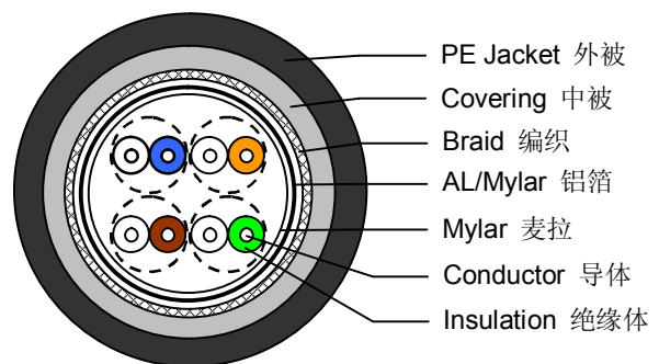
SFTP 线材结构图
