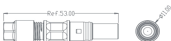
Mini female connector
