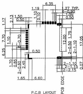
P.C.B LAYOUT TOP VIEW \pm 0.05
