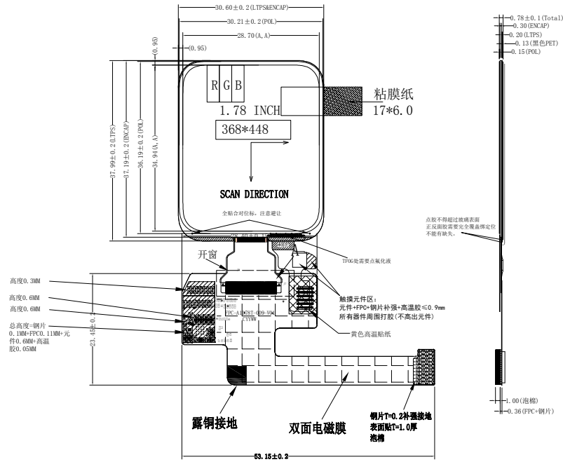
正视图
