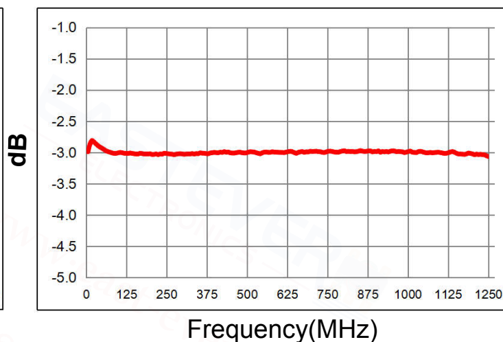
Main line Loss(pin3-4):
