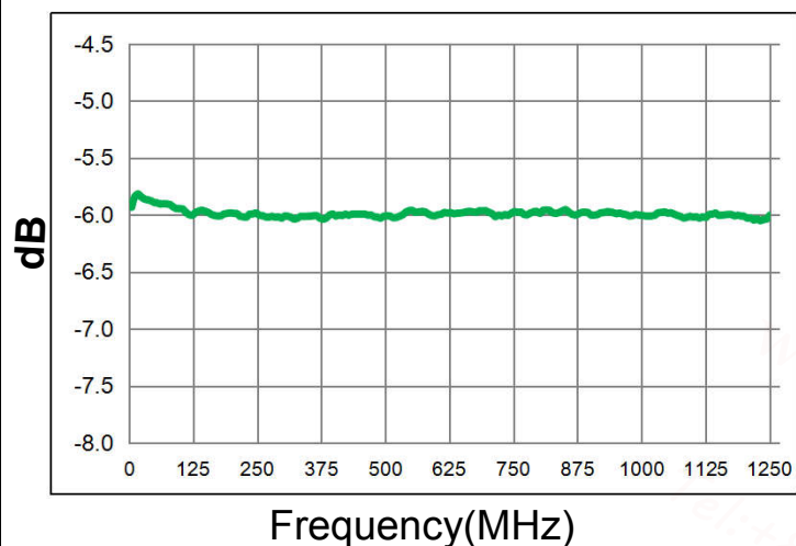
Coupling(pin3-1):
