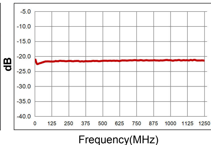
Isolation (Pin1-4)
