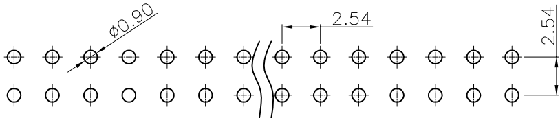
P.C.B LAYOUT
