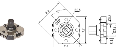
B1724A /B Tact switch 12V 0.05A A : 3.15mm B : 3.85mm
