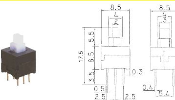
B1719F Tact switch 12V 0.05A F : 5.0mm
