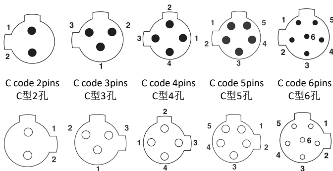
C code 2pins C型2孔 C code 3pins C型3孔 C code 4pins C型4孔 C code 5pins C型5孔 C code 6pins C型6孔
