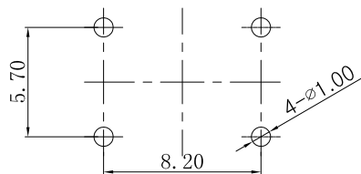
PCB Layout(Pattern Side)
