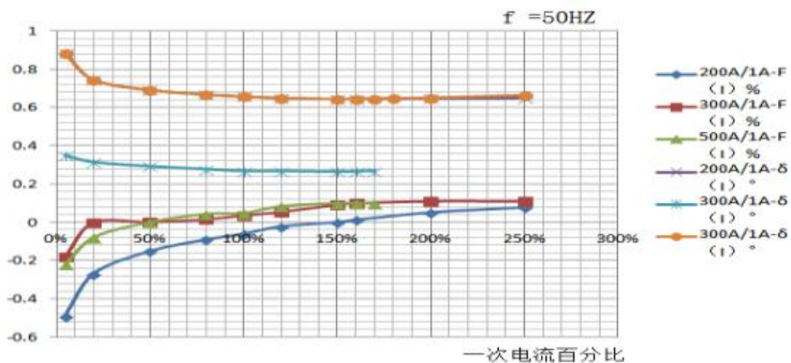
[ SCT0036输出1A, 性能曲线 (1.5平方皮线留长2.5米) ]
