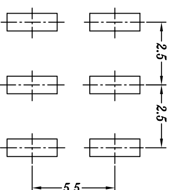
P.C.B LAYOUT
