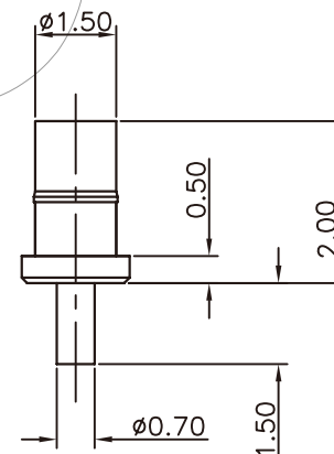
POGO PIN
