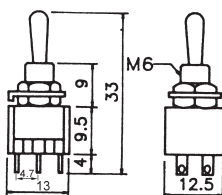
B068F 6P mini toggle switch W/cap (DPDT) on-off-on gold-pin 120V 5A (250V 2A)
