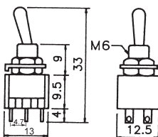
B068E 6P mini toggle switch W/cap (DPDT) on-on gold-pin 120V 5A (250V 2A)
