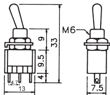
B068B 3P mini toggle switch W/cap (SPDT) on-on gold-pin 120V 5A (250V 2A)
