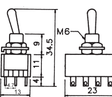
B068L 12P mini toggle switch W/cap (4PDT) on-on gold-pin 120V 5A (250V 2A)
