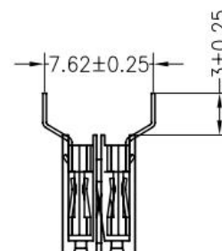
Type02 A=7.62
