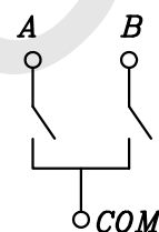
(SW01) 编码回路图
