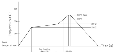
SMT 回流焊
