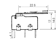
B175GP Mini micro switch PCB terminal (SPDT) on-on 125V 5A (250V 3A) UL
