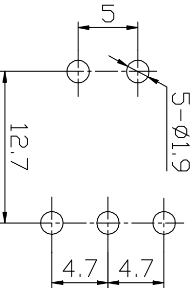
安装尺寸 (Mounting)
