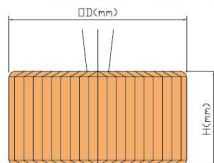
環形變壓器尺寸圖
