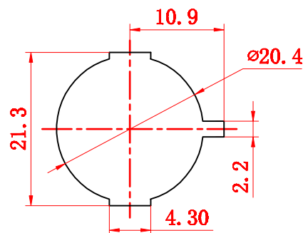
安装尺寸
