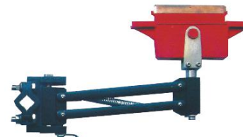
250A集电器 250A Current collector
