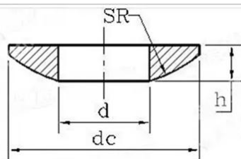
GB849 球面垫圈
