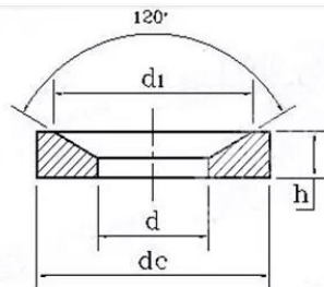
GB850 锥面垫圈
