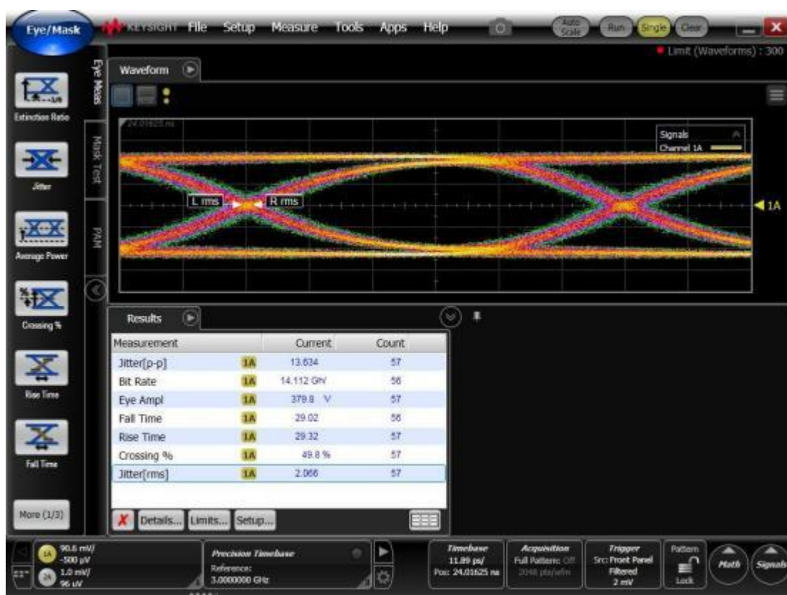
BERTWave E415B 设备 14.025G、PRBS31 码型 眼图
