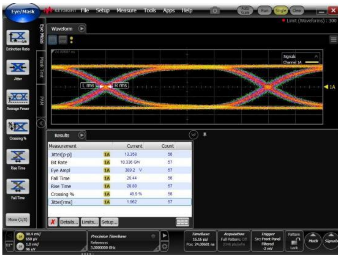
BERTWave E415B 设备 10.3125G、PRBS31 码型 眼图
