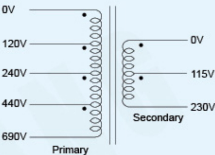
原理图 Schematics
