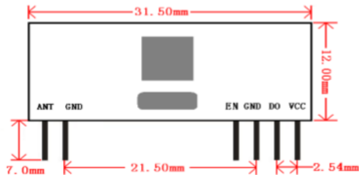
CY08 Dimension
