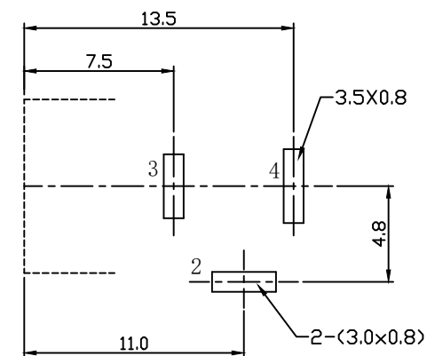
线路板开孔尺寸 P.C.B LAYOUT
