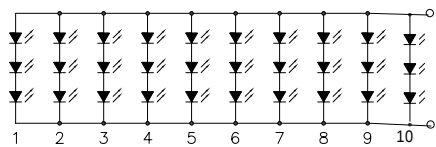
LED 电路图
