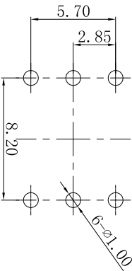
PCB Layout(Pattern Side)
