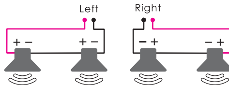
4 ohm
