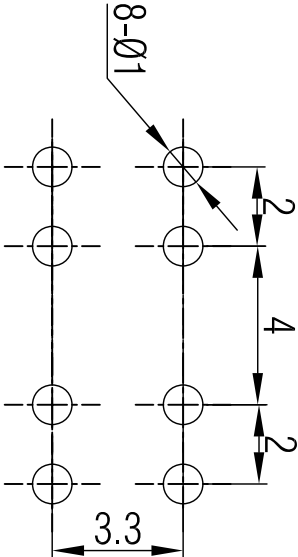
P.B.LAYOUT DIMENSION
