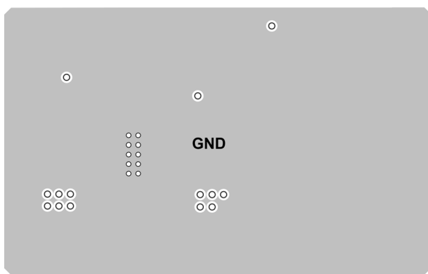
Inner Layer 2
