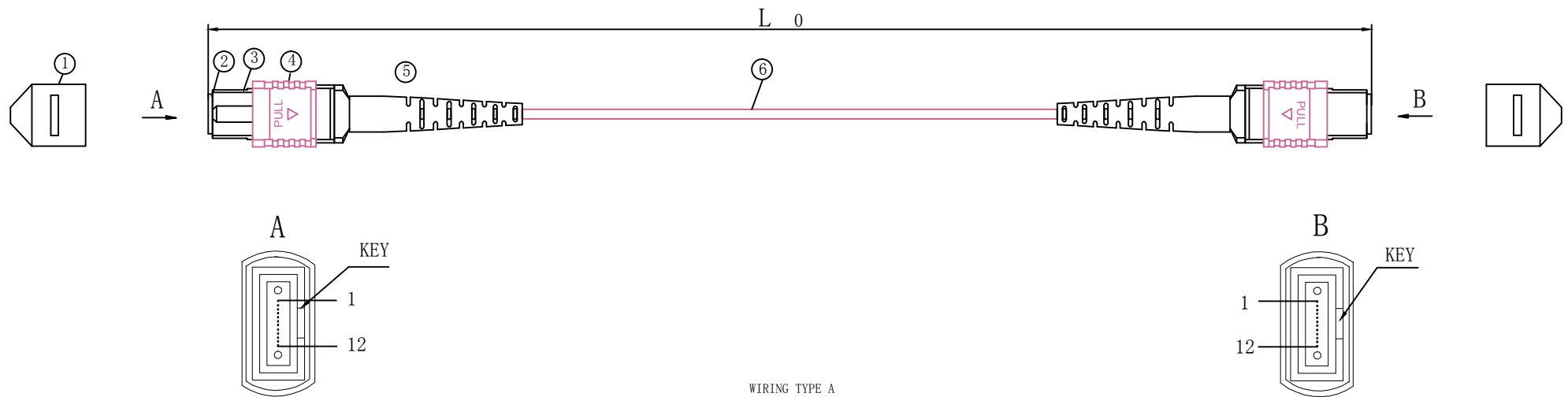
WIRING TYPE A
