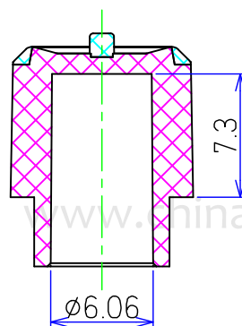
A-A剖视图
