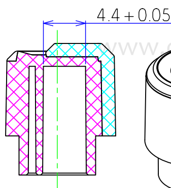
B-B剖视图
