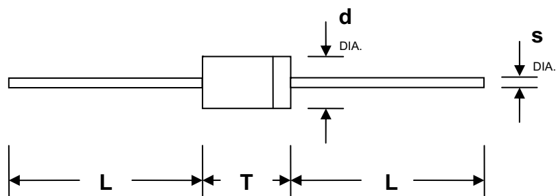
DO-204AC/DO-15
