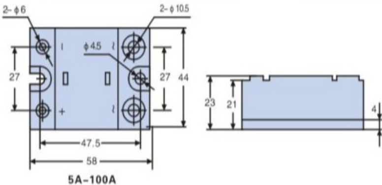
外形尺寸 Dimentions:
