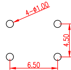
PCB. 焊接图
