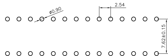
P.C.B LAYOUT
