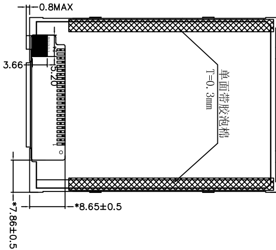
FPC 弯折示意图 展开出货
