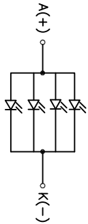
背光电路图 (CIRCUIT DIAGRAM)
