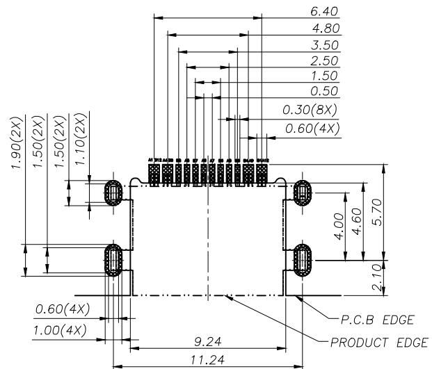
P.C.B LAYOUT
