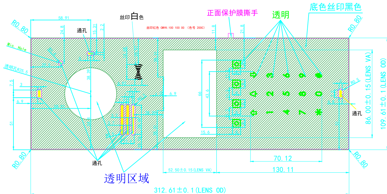
正视图
