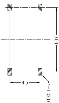
P.C.B. LAYOUT
