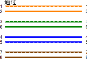
接线图 (T568B)
