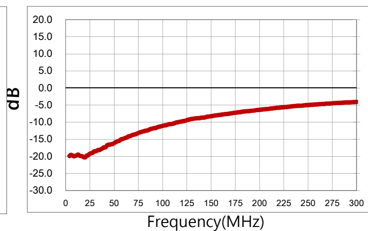
Sdd22
